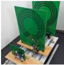
電力を安定供給する ワイヤレス給電装置
