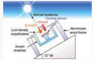
電気無用の冷却デバイス
